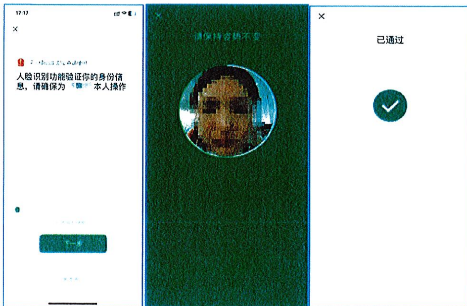
图 1.1-4 人脸识别
